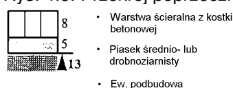
Rys. 4.3. Przekrój poprzeczny nawierzchni na wjeździe z betonowej kostki brukowej
