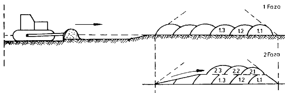
Rys. 1. Schemat zdjęcia ziemi urodzajnej za pomocą spycharki z przesunięciem jej na zwąły (wg S. Datka, S. Lenczewski: Drogowe roboty ziemne, WKŁ 1979)
