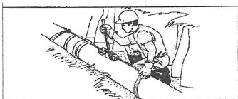
6. Dla mniejszych średnic łączenie wykonuje się ręcznie, dla większych średnic można używać stalowego pręta jako dźwigni, zabezpieczając koniec rury drewnianym klokiem.
