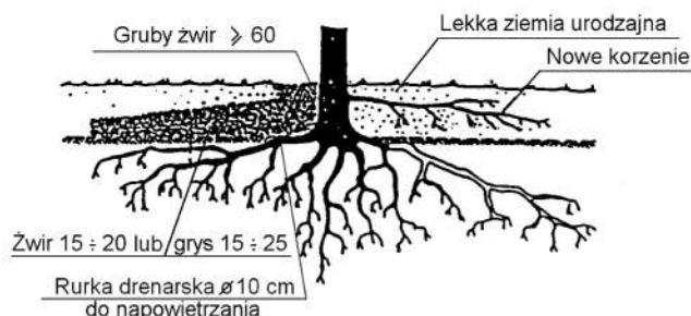
Rys. 4. Pień drzewa obsypany na wysokość 0,2 \pm 0,5 m ze specjalnymi napowietrzającymi warstwami zwirowymi (wg [10])
