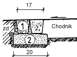
Rys. 3.3. Obramowanie wjazdu z dwóch rzędów kostki kamiennej
