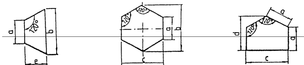
Rysunek 1. Kształt płyt betonowych
