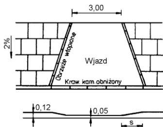
Rys. 3.2. Obrzeże wtopione jako obramowanie wjazdu
