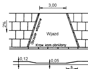
Rys. 3.2. Obrzeże wtopione jako obramowanie wjazdu
