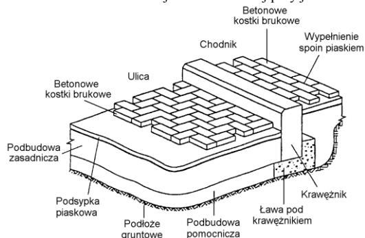
Rys. 1. Widok chodnika z betonowej kostki brukowej przy jezdni oddzielonej krawężnikiem
