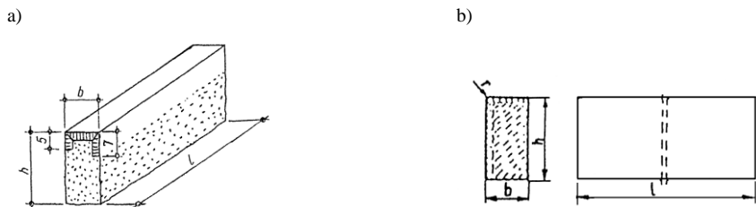
Krawężnik rodzaju A (z wyrównaniem krawędzi)
