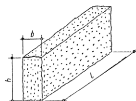
Krawężnik rodzaju B (o powierzchniach surowych)
