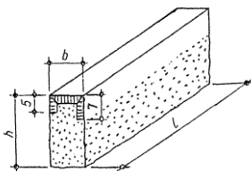
Krawężnik rodzaju A (z wyrównaniem krawędzi)
