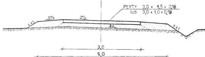
Rys. 5. Przykładowy przekrój poprzeczny nawierzchni z płyt
