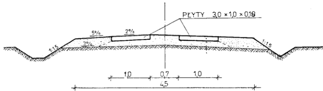
Rys. 4. Przekrój poprzeczny drogi jednopasowej
